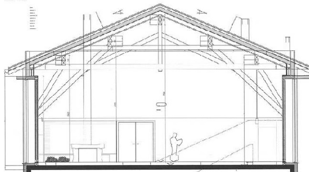
SCHNITTANSICHT A-A Met. 1:50
