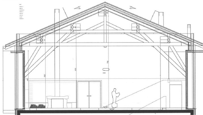
SCHNITTANSICHT A-A Mst. 1:50
